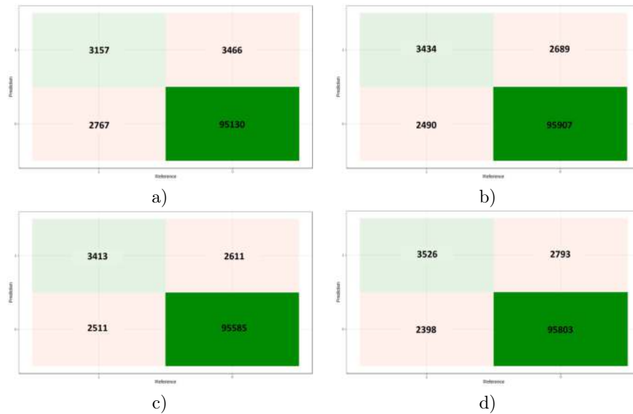
FIGURE 5.6 – Matrice de confusion pour a) GLMNET b) RF c) XGBOOST d) AGGREGATE sur l'échantillon test.
